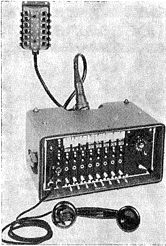
Uudentyyppinen 8-johdon kenttäkeskus. Tällaisia yhdistämällä voidaan muodostaa suurempia keskuksia.
