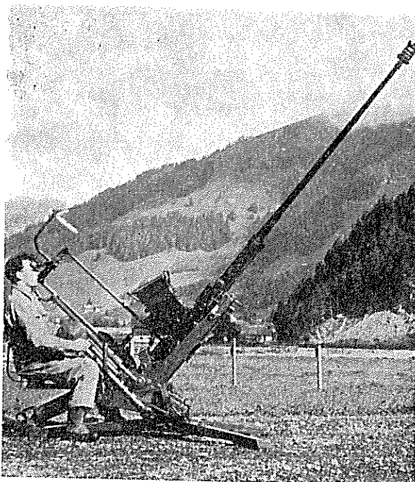
20 MM IT KANUUNA, MALLI 6 ILa/5TG
