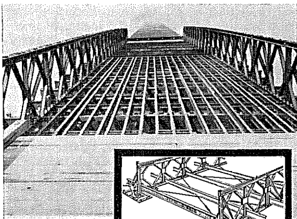
BAILEY BRIDGE ELEMENTTISILTA
