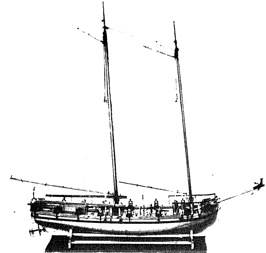
Ruotsalainen tykkiparkassi 1700-luvun lopulta. Pituus 16 m, leveys 4 m, 8 airoparia, 40 miestä. Aseistus: 1 kpl 12–24-naulan kanuuna ja 16 kpl 2–3-naulan nikhakoja. (Pienoismalli Tukholman merihistoriallisessa museossa)
