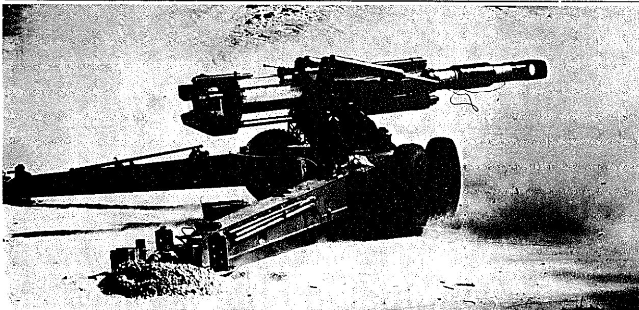
Tämä Tampellan valmistama kenttätykki 155 K/68 on alusta loppuun kotimaista työtä.
