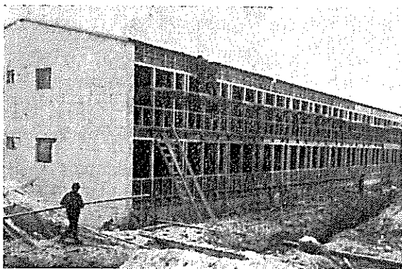
Sodankylään kohoava asuntotalo
