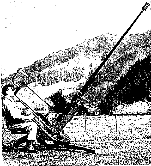
20 MM IT KANUUNA, MALLI 6 ILa/5TG
