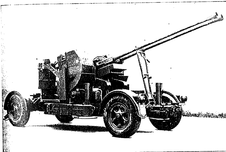
TUTKAOHJATTU KAKSOISILMATORJUNTAKANUUNA, MALLI, 2 ZLa/353
