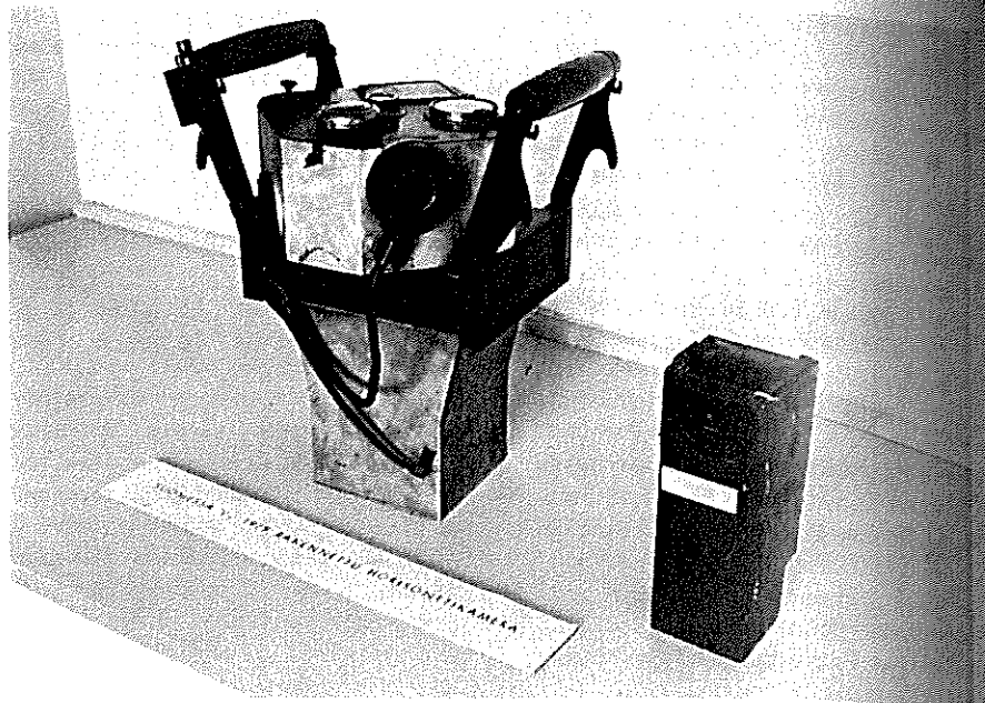
Museon harvinaisuuksia on kenr Nenosen 1928 suunnittelema ja asevarikolla valmistettu horisonttikamera, joka paransi merkittävästi lentokuvauksin suoritettua kartoitus toimintaa.
