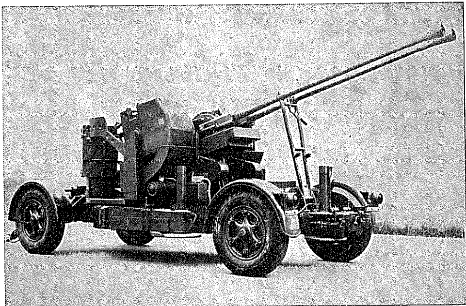
35 mm tutkaohjattu kaksois-ittykki, malli 2ZLa/353
